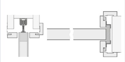
Skizze Variante B: Schiebetürzarge in Wand
