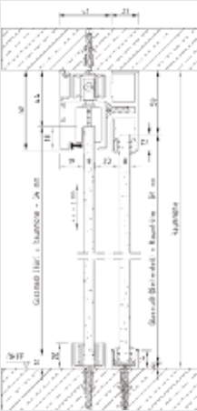
Sturz-/Zwischen-Wand-Montage mit festem Seitenteil (zu 5802 16)
